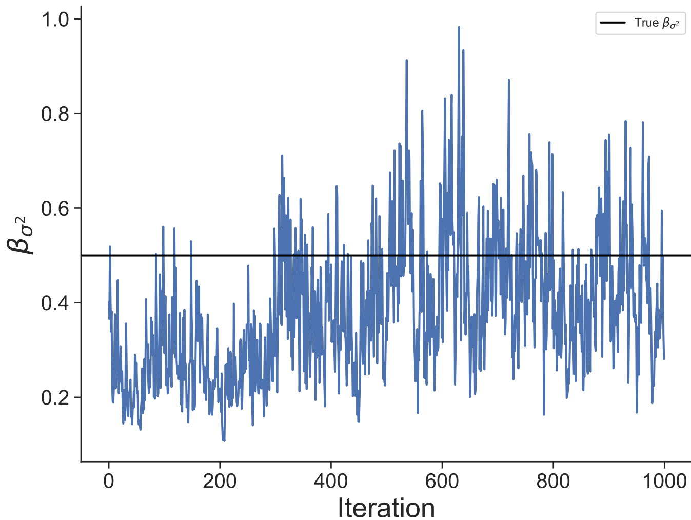
Dataset 25
