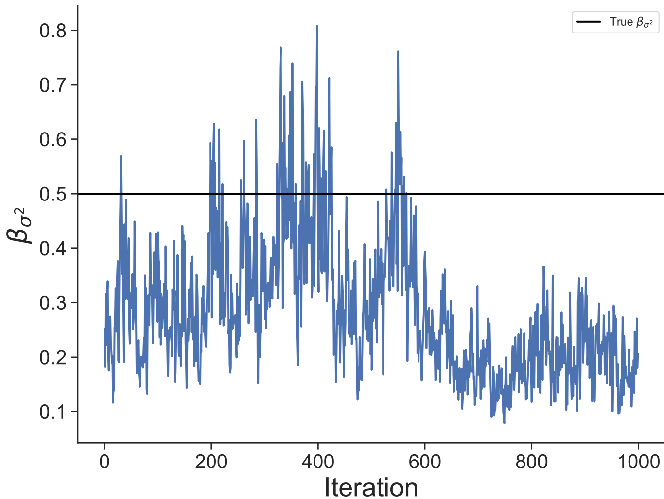
Dataset 22
