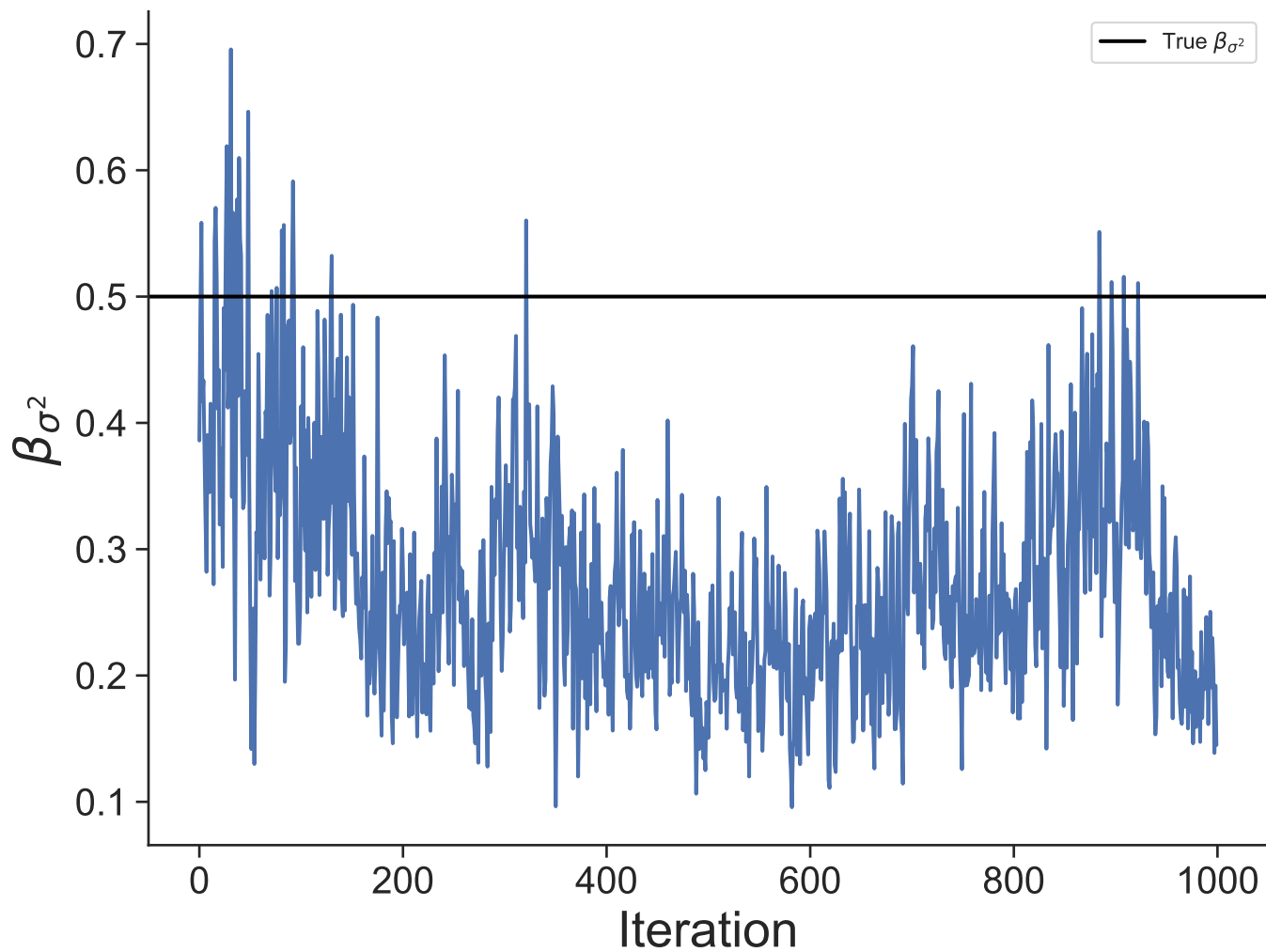
Dataset 5
