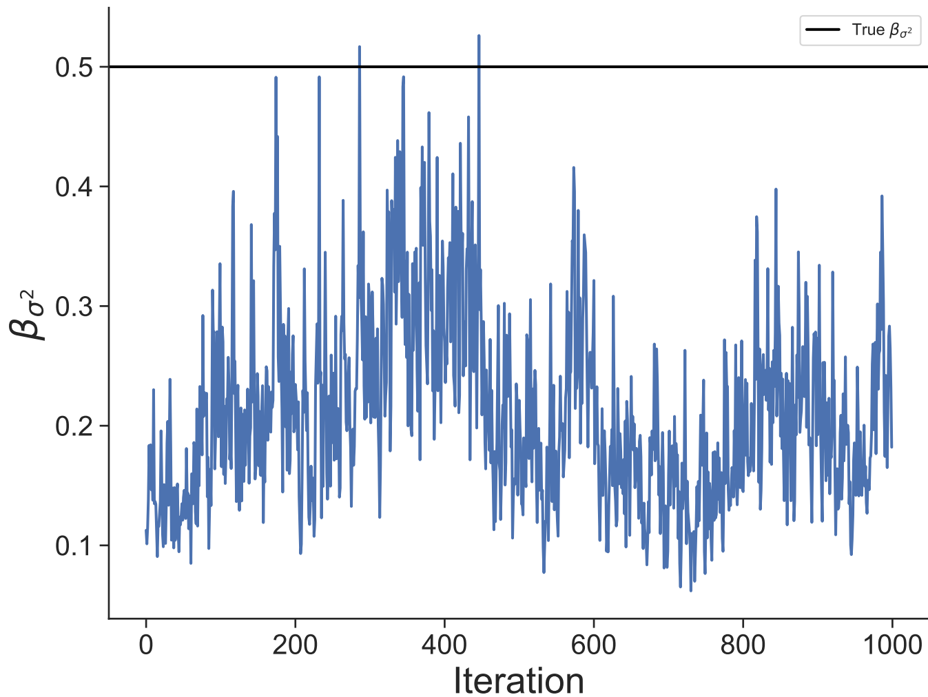
Dataset 34
