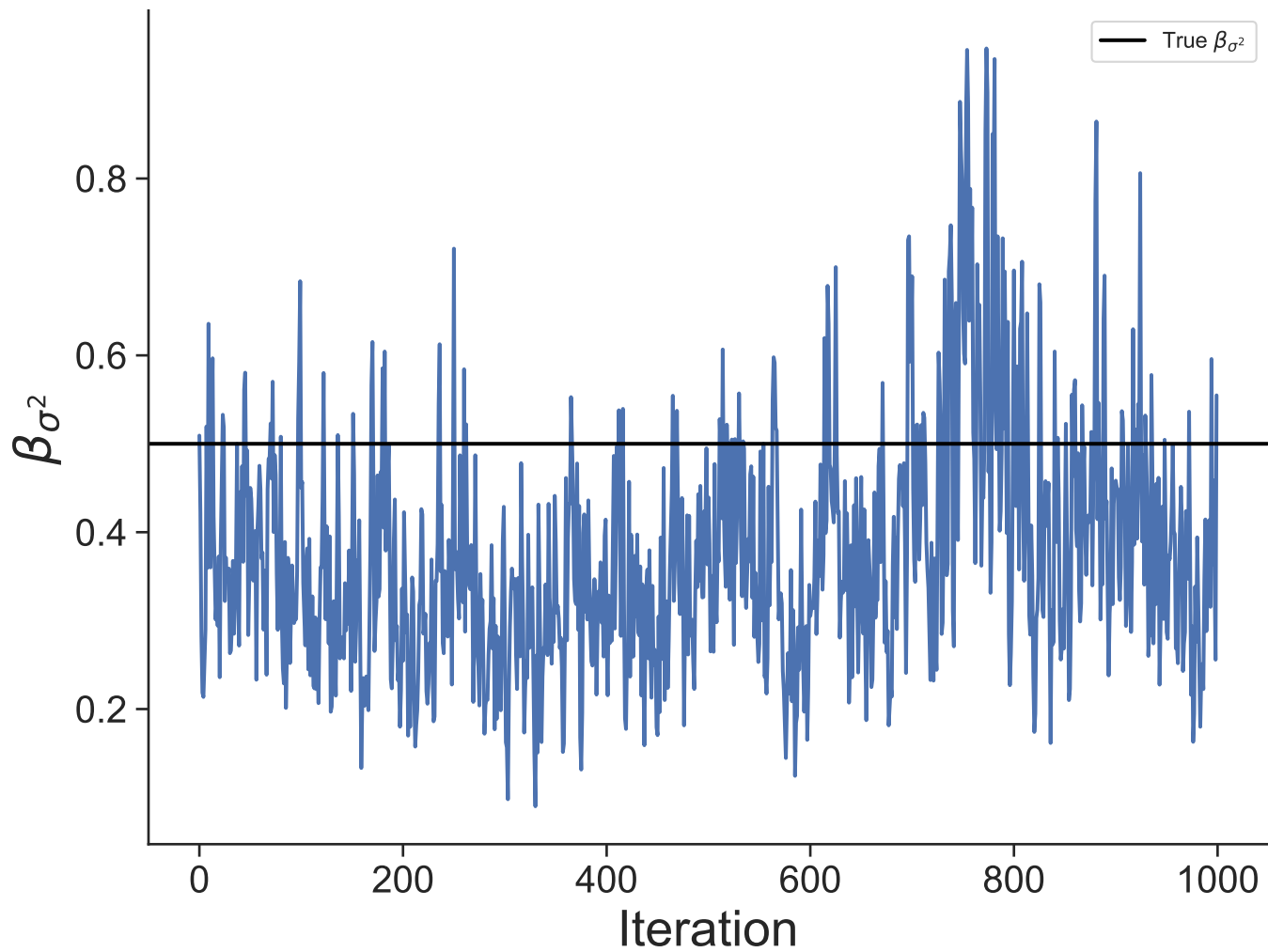
Dataset 15
