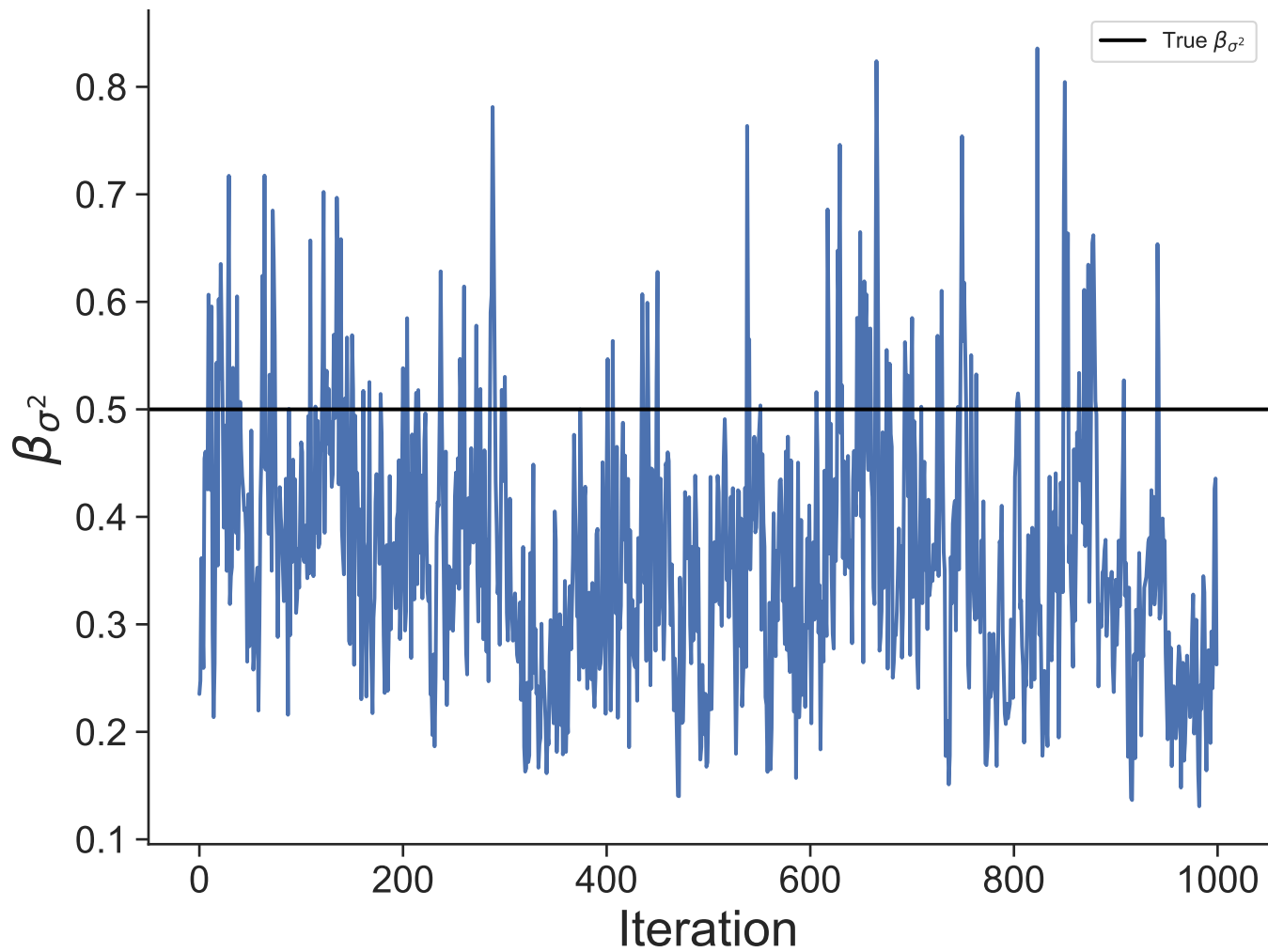
Dataset 16
