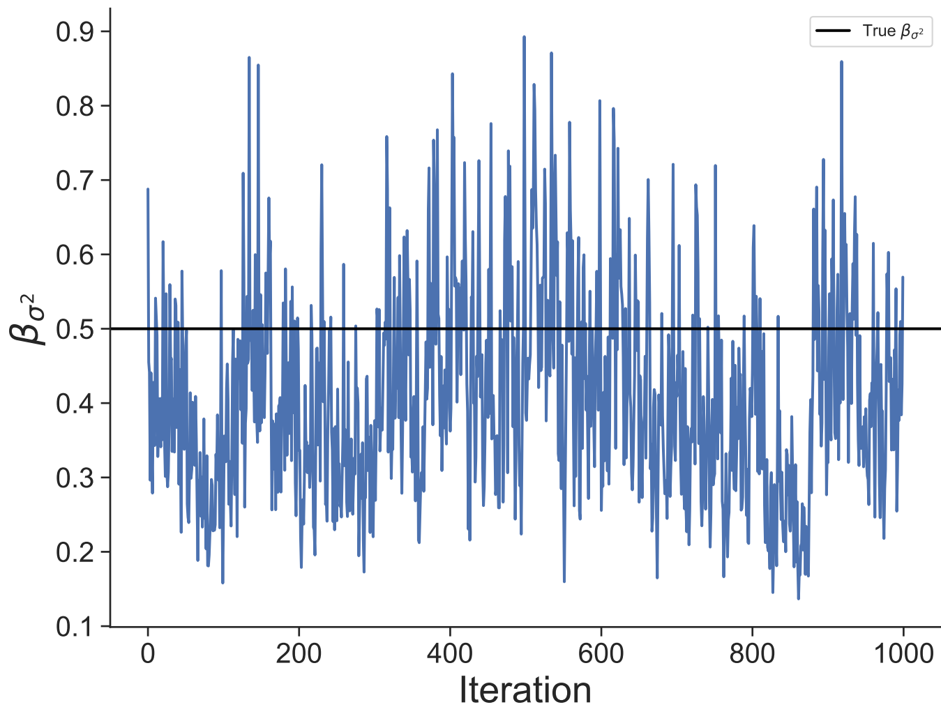
Dataset 35
