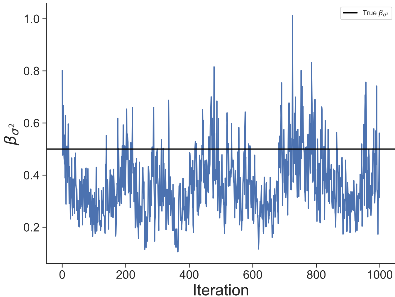
Dataset 46
