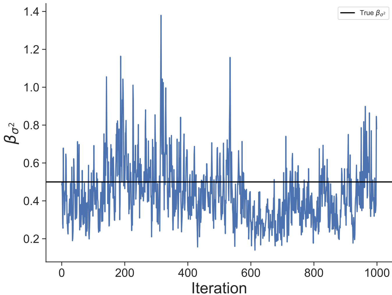
Dataset 26
