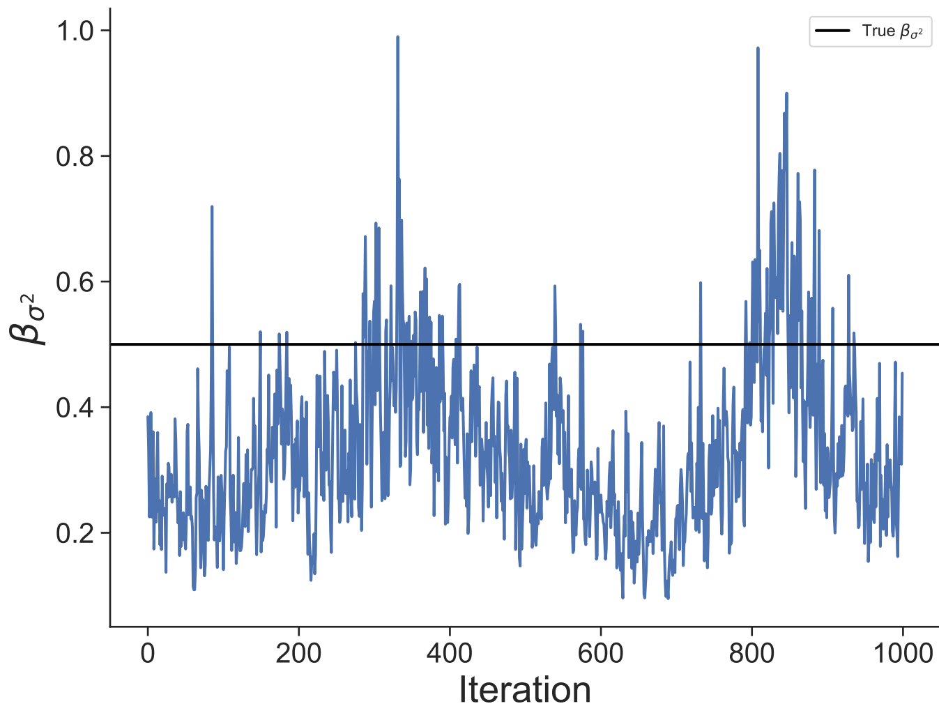
Dataset 37
