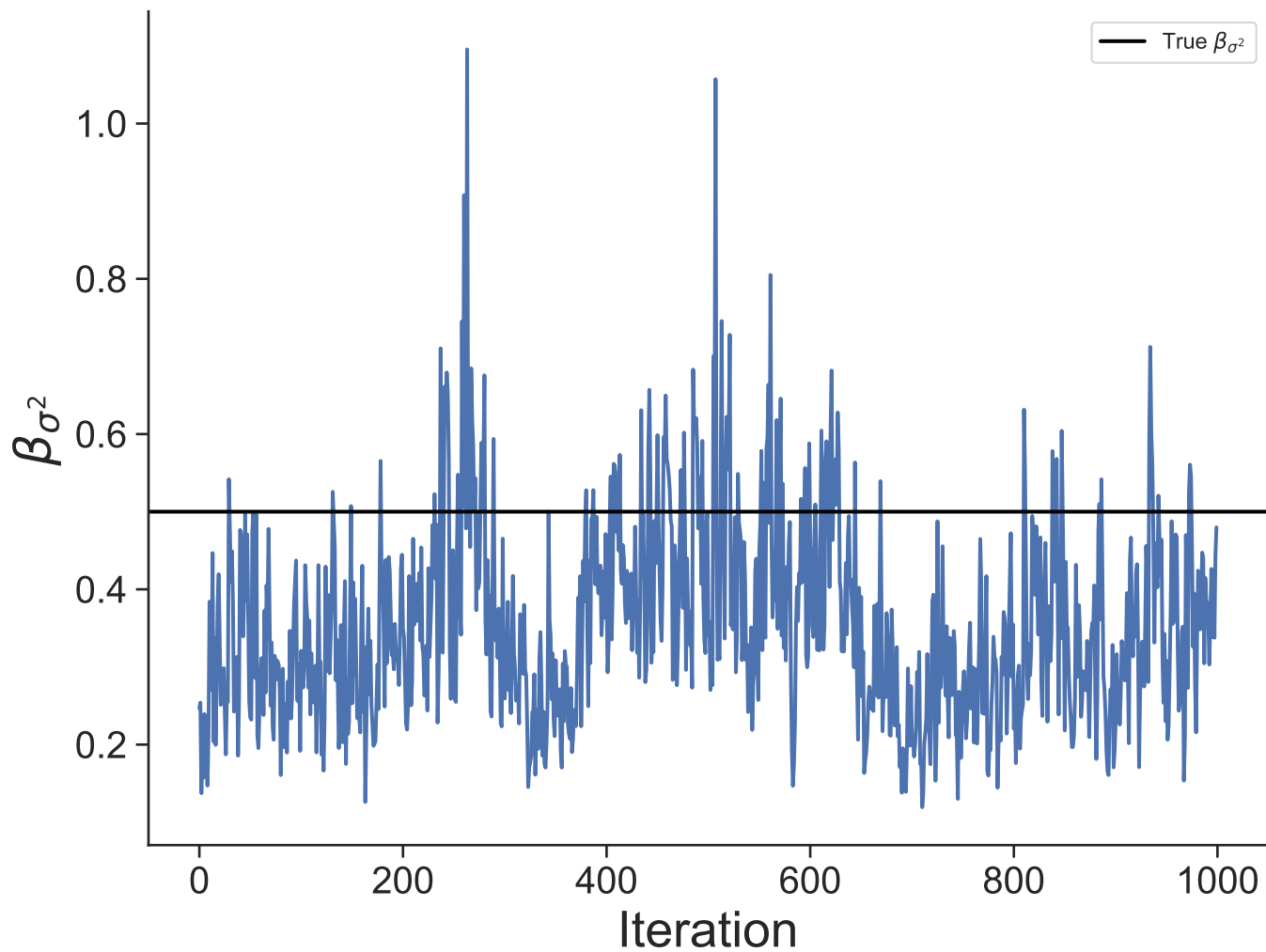
Dataset 38
