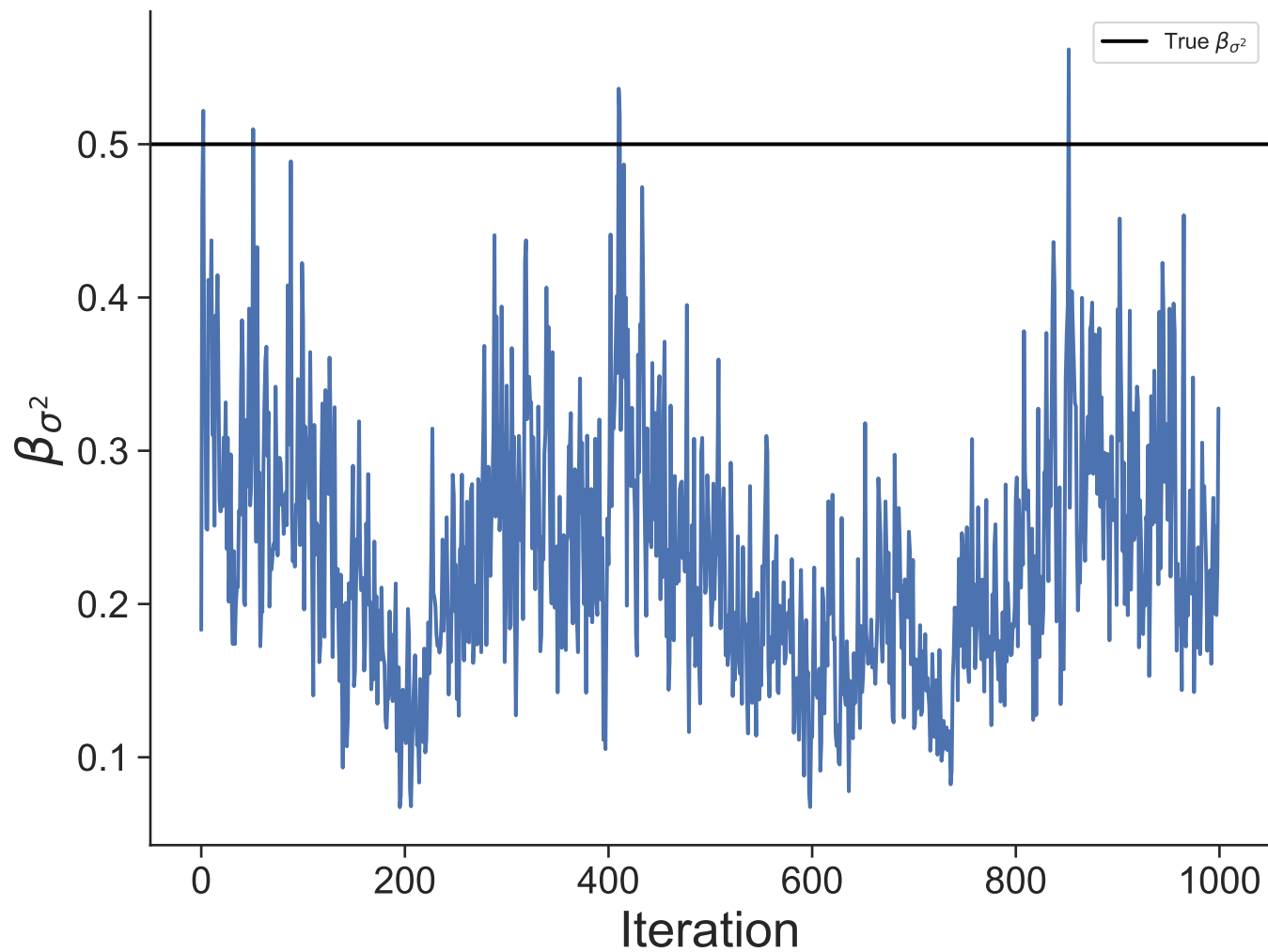
Dataset 42
